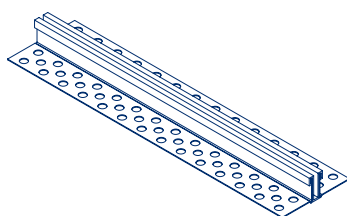
axonométrie échelle 1:5
