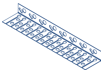
axonométrie échelle 1:5
