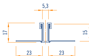
vue frontale échelle 1:2
