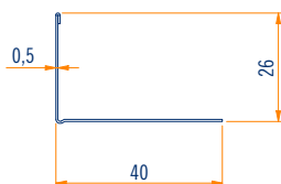
vue frontale échelle 1:2
