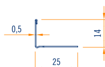
vue frontale échelle 1:2
