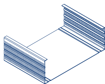
assonometria scala 1:5
