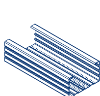
assonometria scala 1:5
