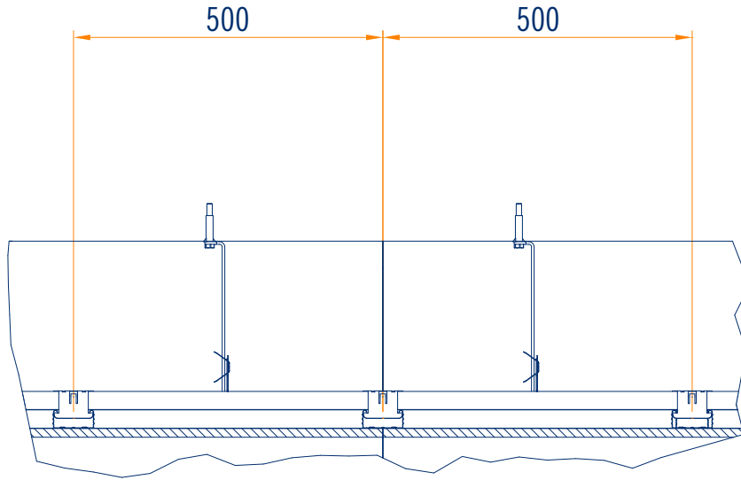
sezione B-B (1:10)
