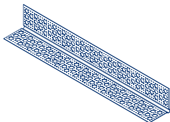
assonometria scala 1:5
