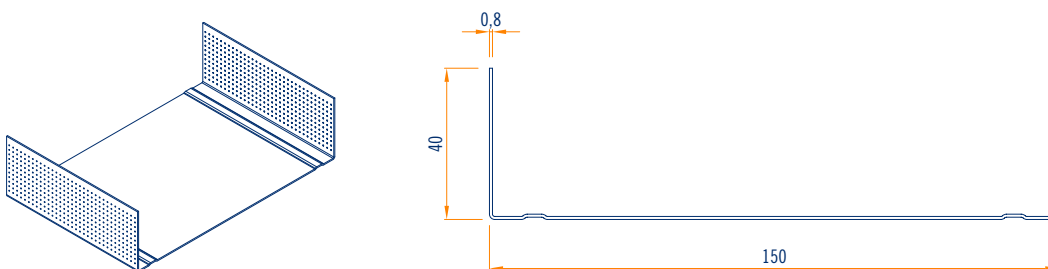
assonometria scala 1:5
