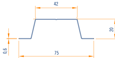
vista frontale scala 1:2
