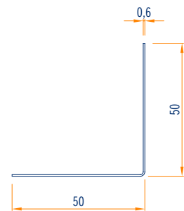
vista frontale scala 1:2
