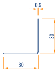
vista frontale scala 1:2
