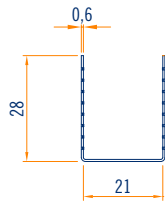
vista frontale scala 1:2
