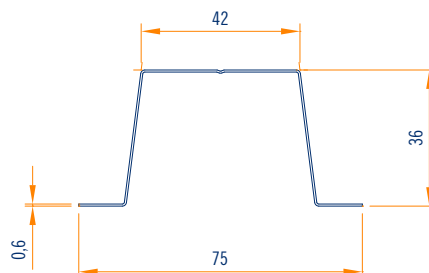
vista frontale scala 1:2
