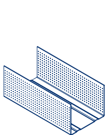
assonometria scala 1:5
