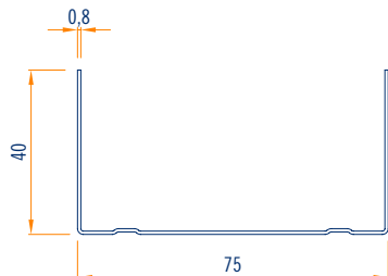
vista frontale scala 1:2
