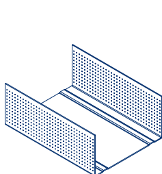
assonometria scala 1:5
