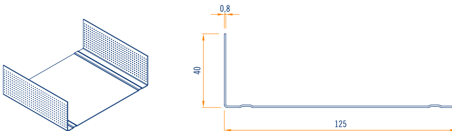
assonometria scala 1:5
