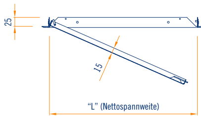
Maßstabschnitt (geöffnet) 1:10
