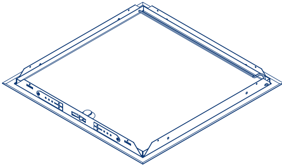
Axonometrie (geschlossen) Maßstab 1:10
