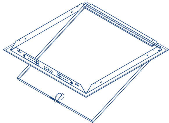
Axonometrie (geöffnet) Maßstab 1:10
